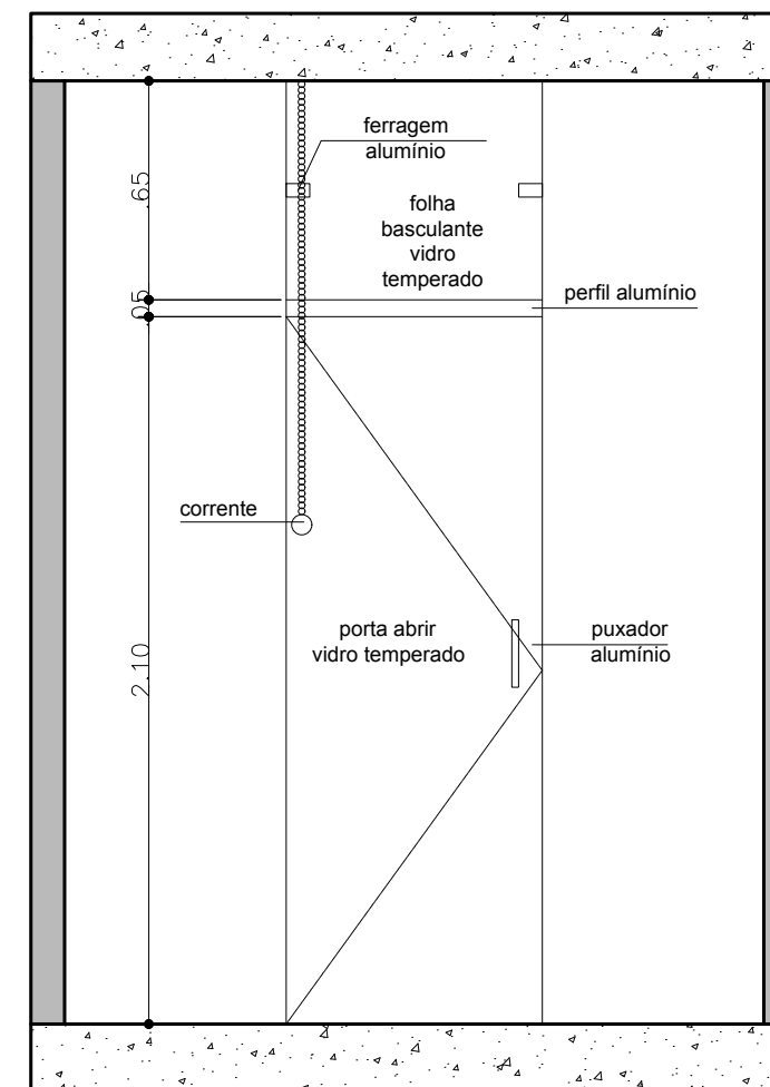
VISTA 2 esc. 1:25
