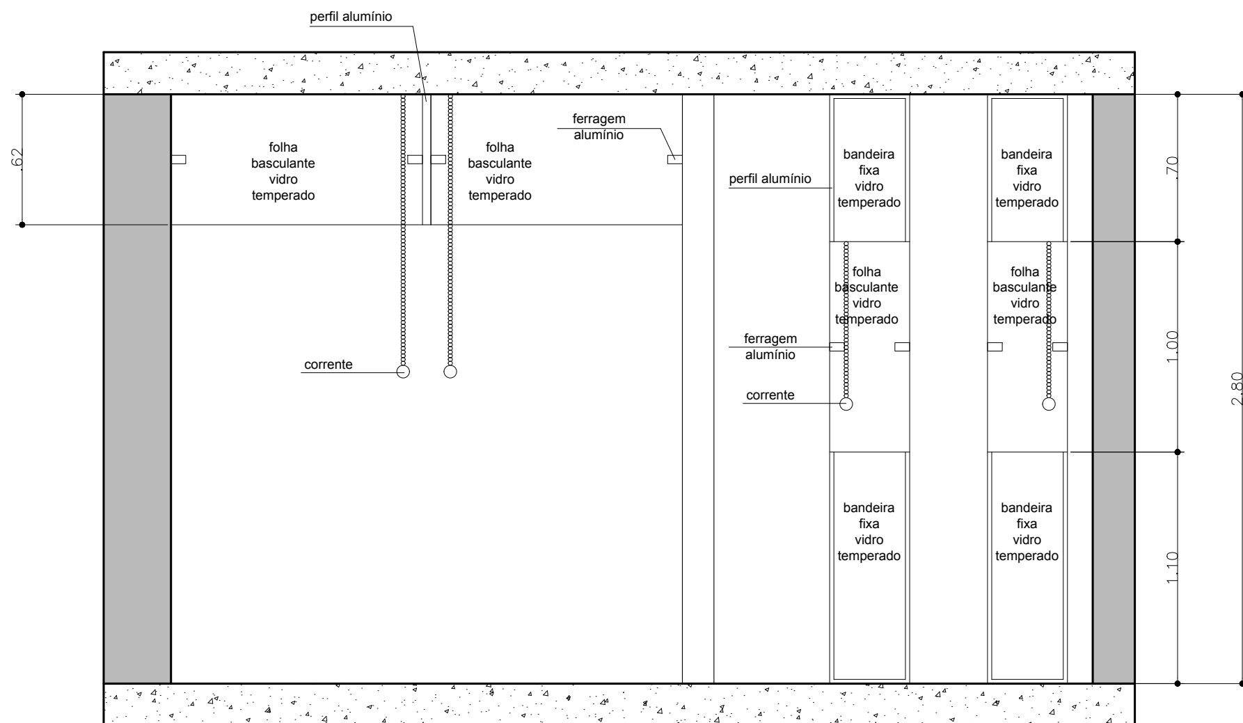
VISTA 1 esc. 1:25
