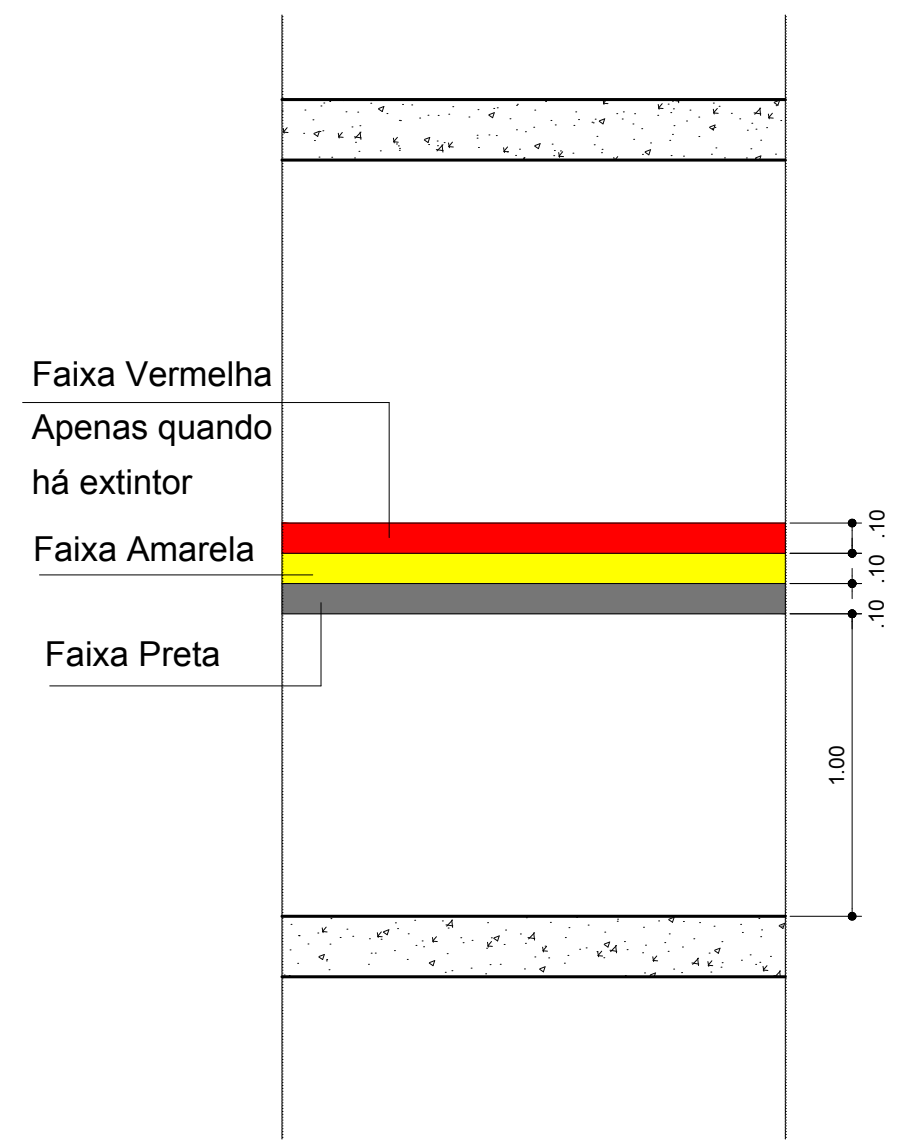
DETALHE 01 PAREDES E PILARES esc 1:25
